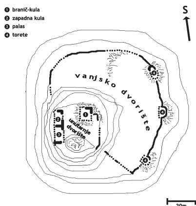
Tlocrtna skica tvrdoga grada Blagaja (prema: < http://jupiter.elte.hu > i Bojanovski, "Blagaj na Sani", 16)
